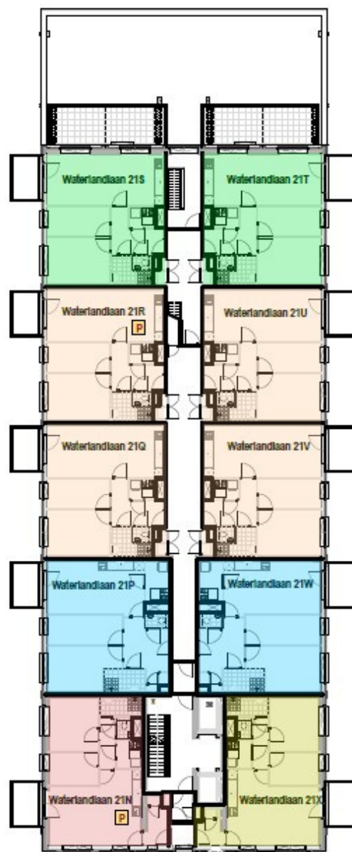
ZESDE VERDIEPING
